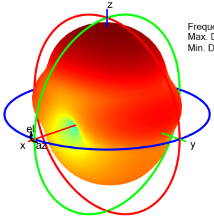
pifa
