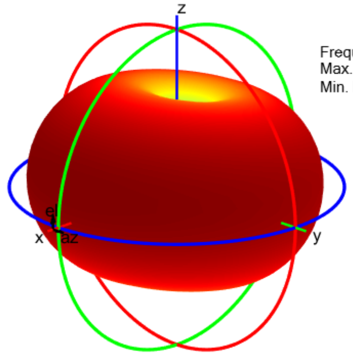
dipoleHelixMultifilar
